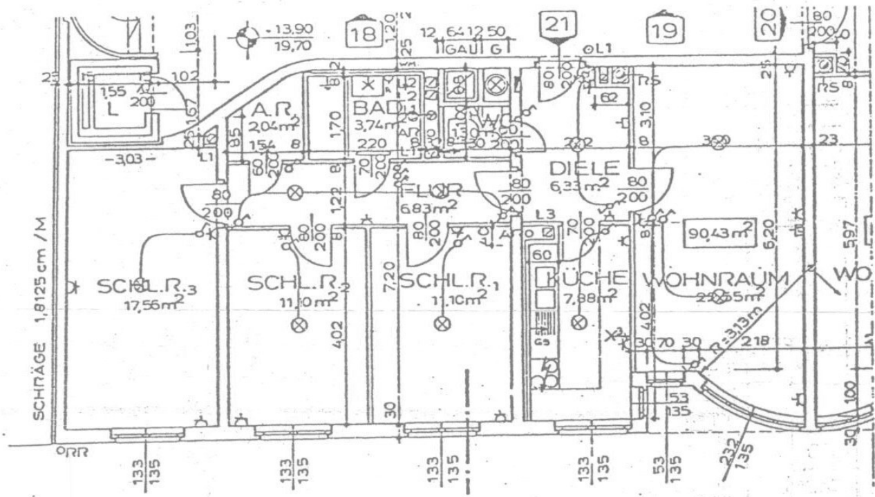
Grundriss Brigittagasse 11/9
